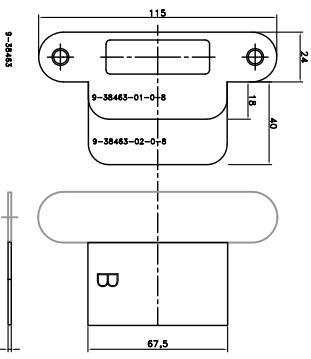
Voorzijzicht sluitplaatlip-inkrozing
