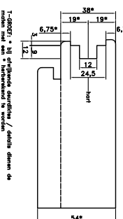
VOORZIJDT DETAIL 2: deurslot 38 / 54 mm T-groef
