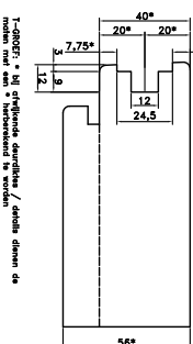
VOORZIJDT DETAIL 4: deurslot 40 / 56 mm T-groef
