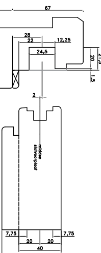
VOORZIJDT DETAIL 3: deurslot 40 / 56 mm Sluitkom-geplaat
