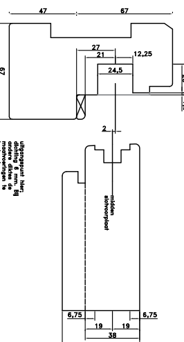
VOORZIJDT DETAIL 2: deurslot 38 / 54 mm T-groef
