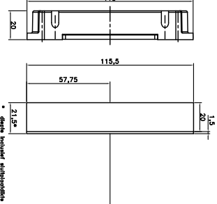
Zijprofiel sluitkom-inkrozing [A]
