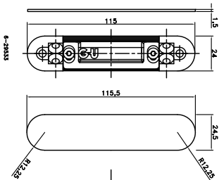
Voorzijzicht sluitkom-inkrozing [B]
